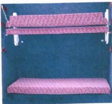
Liegebetten inkl. Drehmechanismus und Auflagen für Liegewagen
